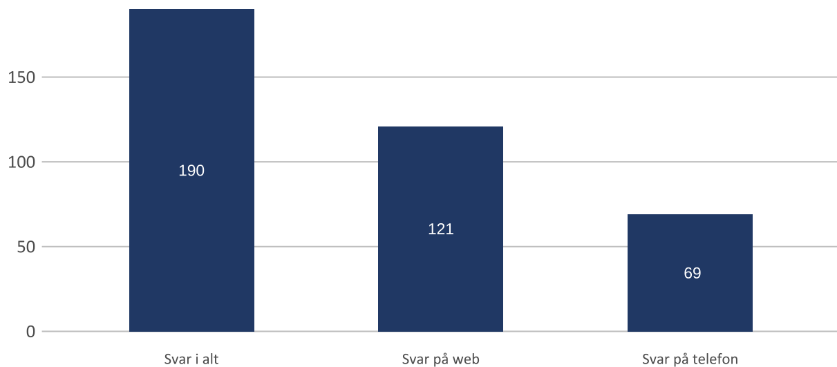
Figur A: Svarene vises for Ishøj Kommune i antal i alt, og for web og for telefonisk interview
