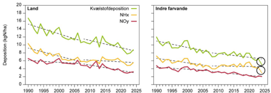
Figur 1.3. Udviklingstendens for deposition af kvælstof til danske landområder og indre danske farvandsområder. Figurene viser den samlede deposition, og deposition opdelt på hhv. NH x (ammoniak og ammonium) og NO y (kvælstofdioxid, salpetersyre og nitrat). NH x stammer primært fra landbrug og NO y stammer hovedsageligt fra forbrændingsprocesser. Stiplede linjer er beregnede lineære regressionslinjer opdelt i perioden fra 1990 til 2007 og 2008 til 2024. Udviklingstendenserne i deposition til landområder er beregnet som middelværdi af måleresultaterne fra Anholt, Tange og Ulfborg i perioden op til 2010. Efter 2010 er Risø inkluderet i udviklingstendensen for derved at øge datarepræsentativiteten. Enkelte manglende delresultater er skønnet f.eks. på basis af sammenligning med andre målestationer (Poulsen et al., 2025).
