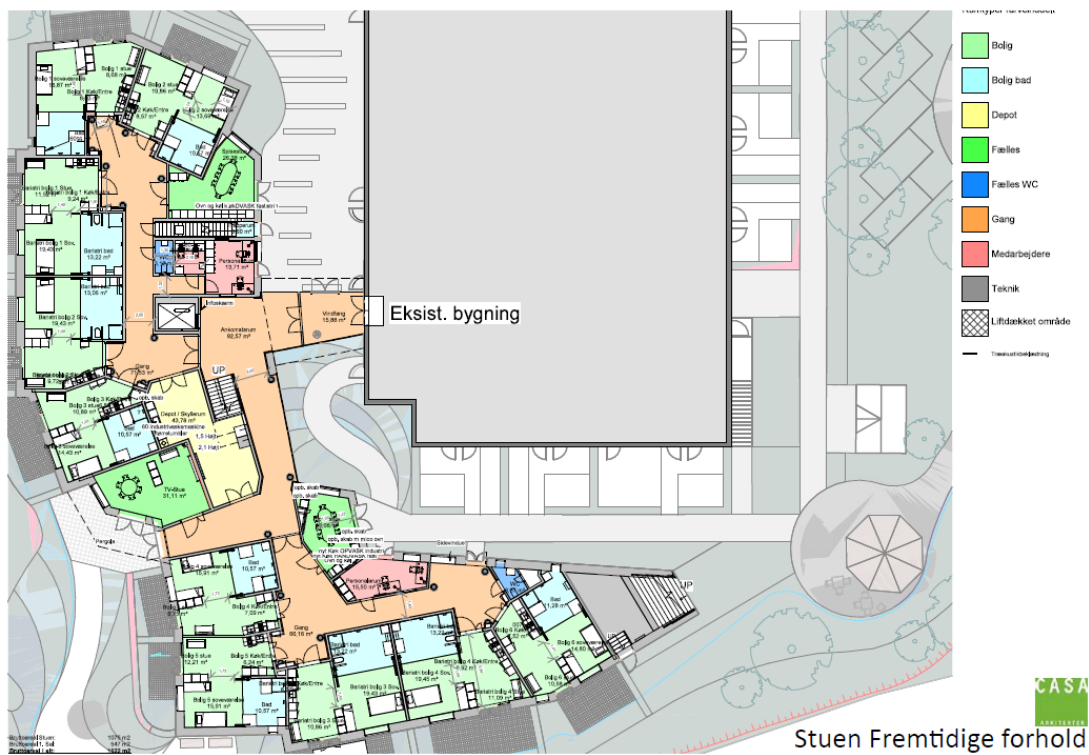
Billede 42. Plantegning fra CASA Arkitekter af den nye bygning i stueplan med lejligheder. Bygningen drejer sig, så indretningen ikke er spejlvendt.
